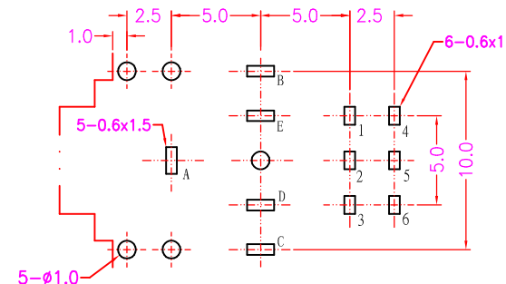
印制板开孔示意图
